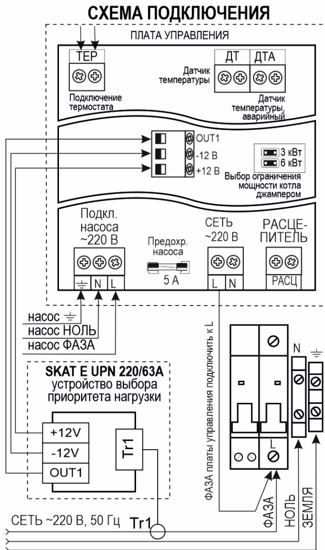
Схема подключения устройства выбора приоритета нагрузки SKAT E UPN 220/63A
